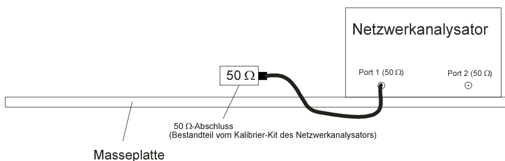
Bild 4 Kalibrieraufbau '50 \Omega ' für Asymmetrische Impedanz und Phasenwinkel
