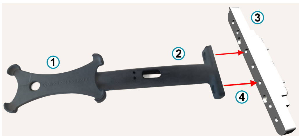
Рис. 7-12: R&S CMQ-B719A опция «Drawer Fixture 2», номер для заказа 1537.6355.02
