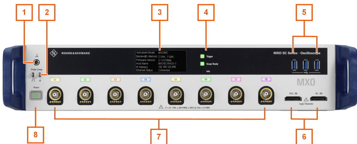
图 4-1: MXO 58C 前视图，具有八路输入通道
