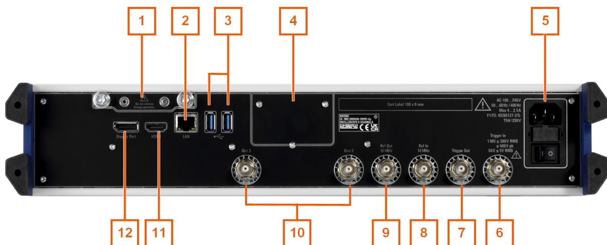
图 4-2: MXO 5C 系列示波器的后面板视图
