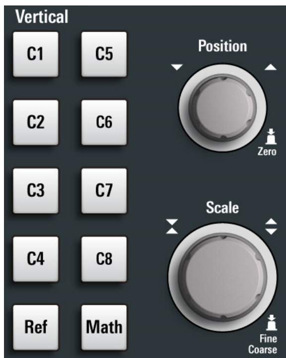
图 5-5: MXO 5 的垂直控件，具有 8 路输入通道
