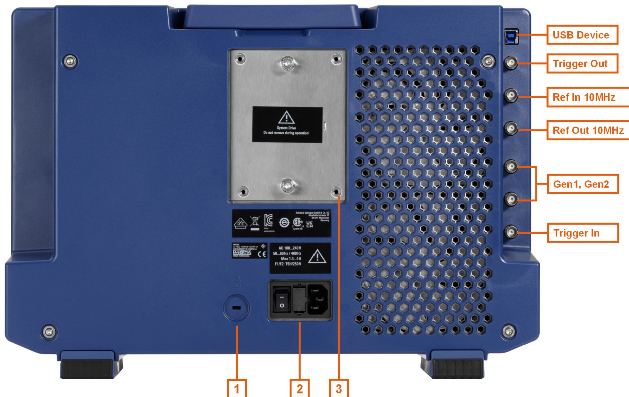
图 5-3: MXO 5 后面板视图
