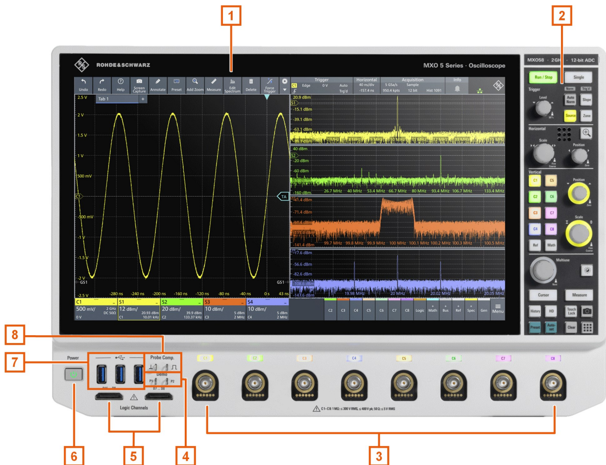
图 5-1: MXO 5 前视图，具有八路输入通道
