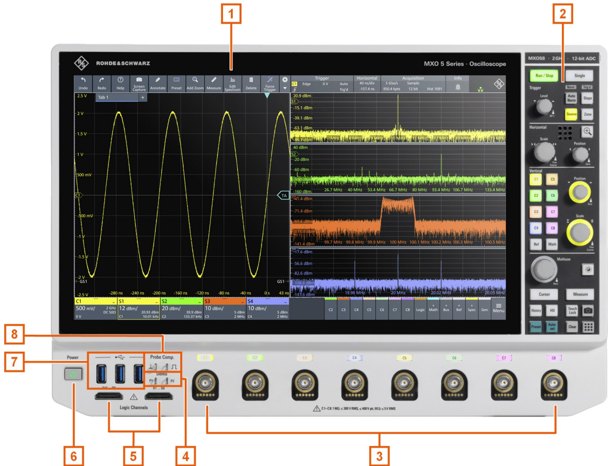
그림 5-1: 8 입력 채널의 MXO 5 전면
