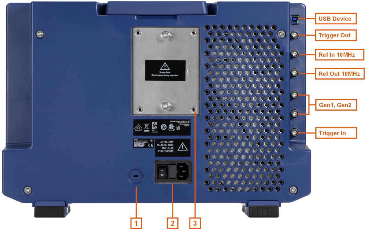
그림 5-3: MXO 5의 후면 패널
