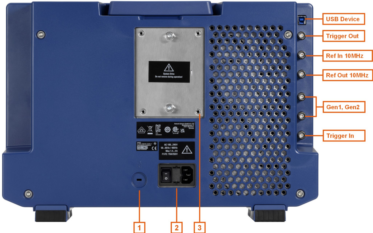
그림 5-3: R&S MXO 5의 후면 패널
