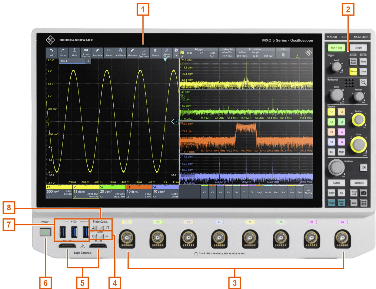
그림 5-1: 8 입력 채널의 R&S MXO58 전면
