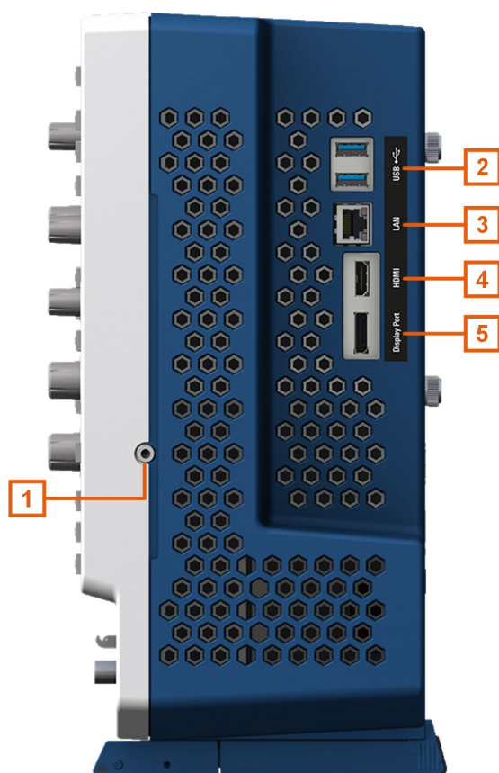
図 5-2: R&S MXO 5 の側面図
