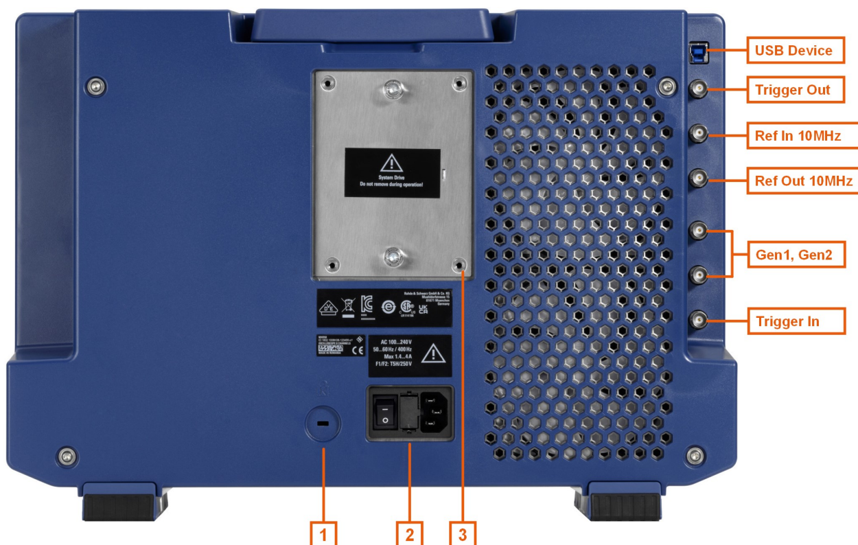
図 5-3: R&S MX0 5 のリアパネル図
