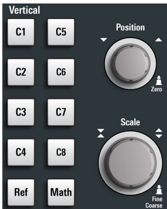
図 5-5: 8つの入力チャンネルを搭載した R&S MXO 5 の垂直軸コントロール
