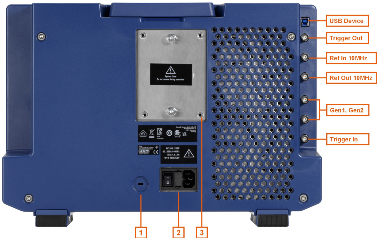
Figura 5-3: Vista del panel posterior del Osciloscopio MXO 5
