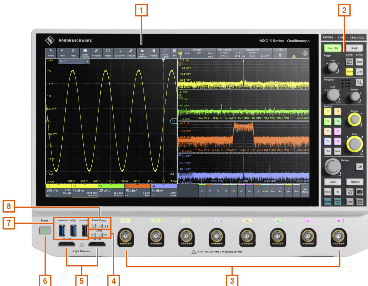
Figura 5-1: Vista frontal del Osciloscopio MXO 5 con 8 canales de entrada
