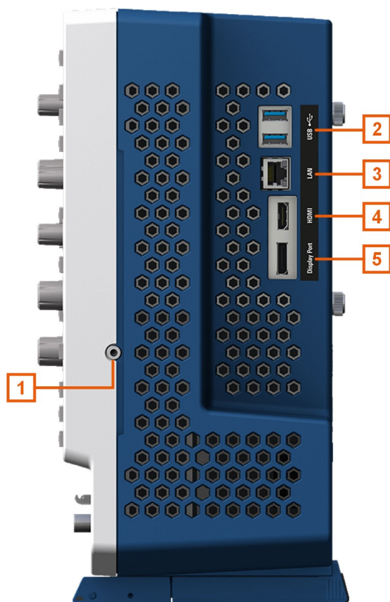
Figura 5-2: Vista del panel lateral del Osciloscopio MXO 5
