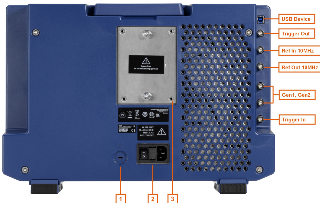
Bild 5-3: Rückseitenansicht des MXO 5
