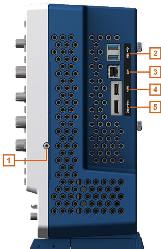
Bild 5-2: Seitenansicht des MXO 5
