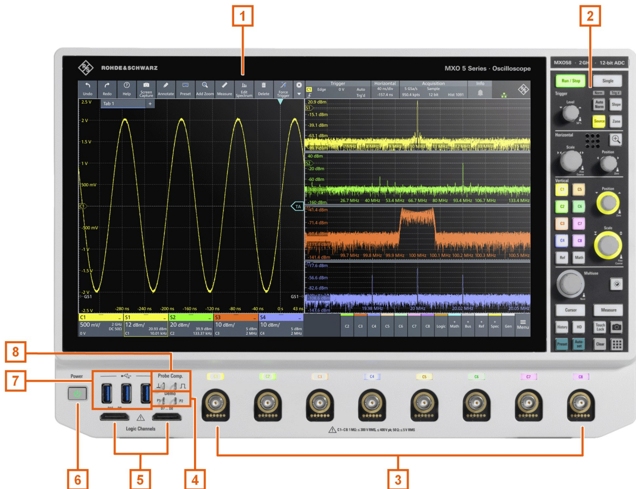
Bild 5-1: Frontansicht des MXO 5 mit 8 Eingangskanälen
