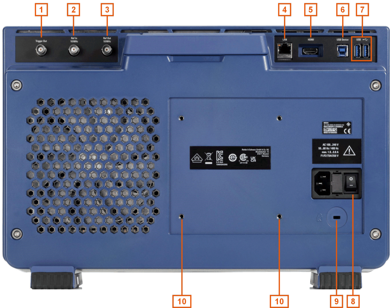
图 5-3: MXO 4 后面板视图
