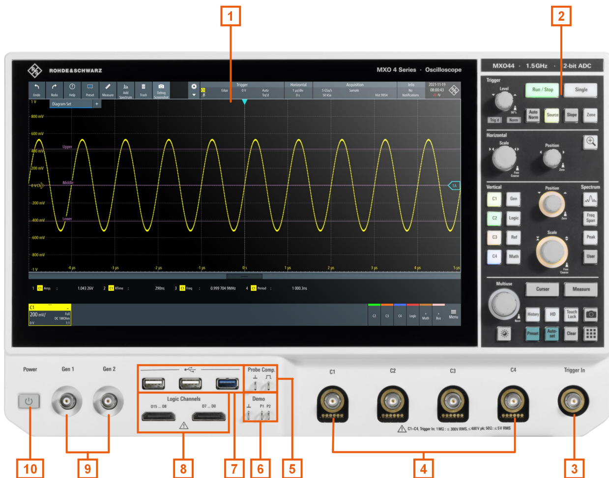
图 5-1: MXO 4 前面板
