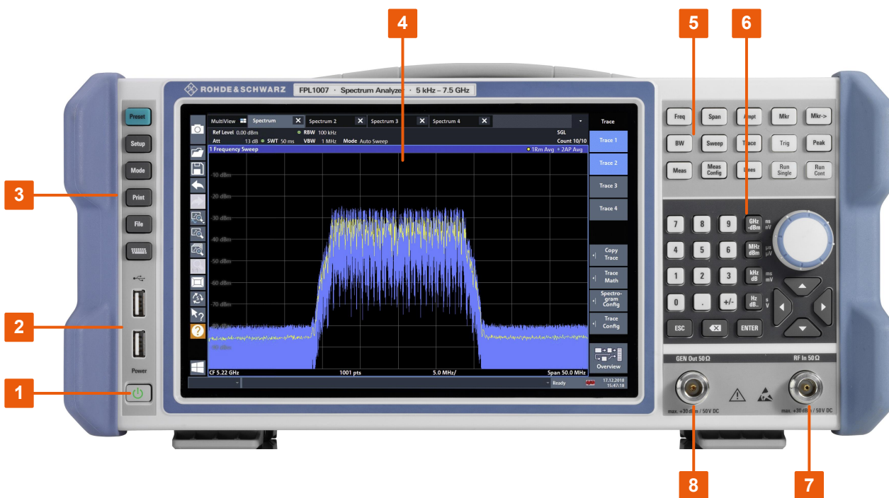
图 5-1: R&S FPL1000 前面板视图
