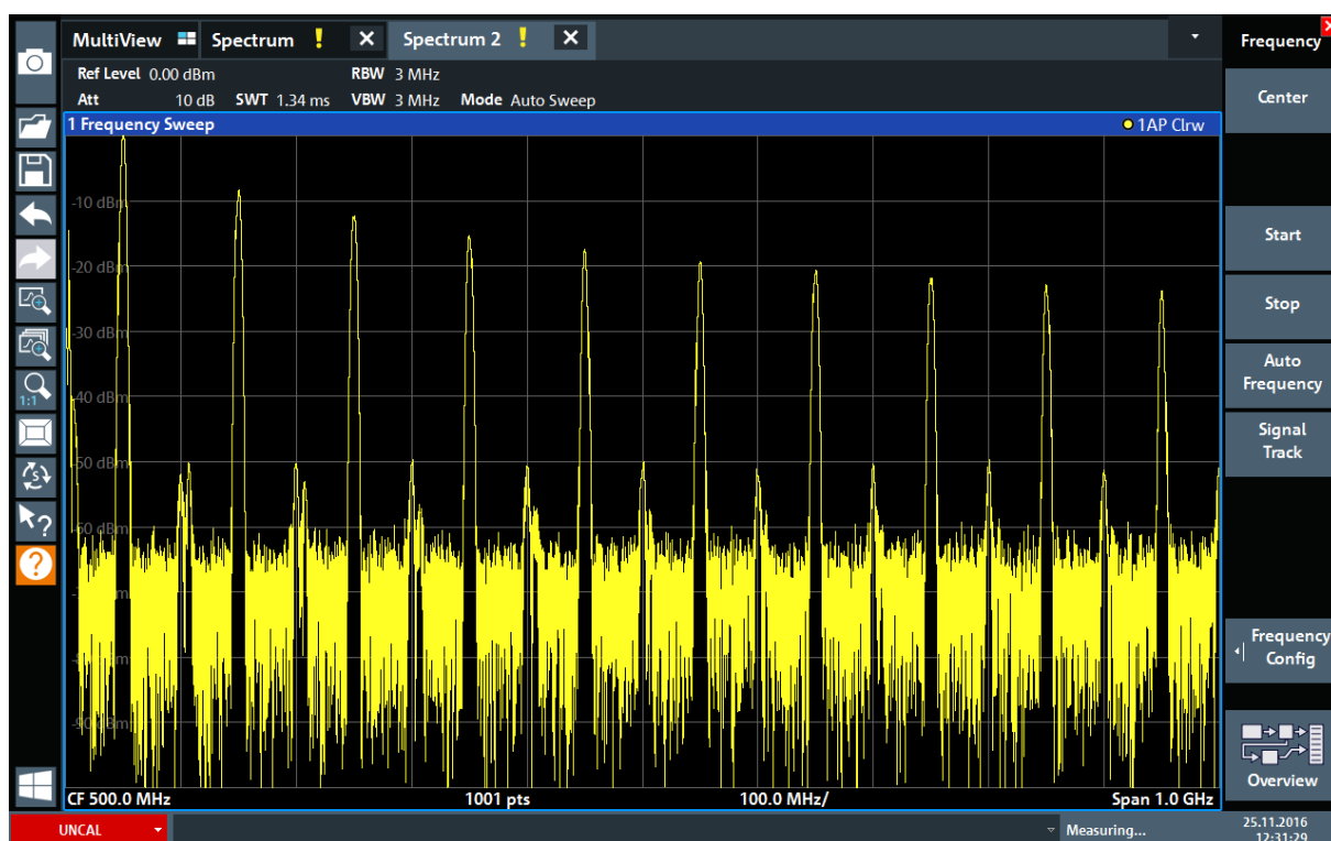
图 6-6: 具有更大频跨的校准信号频谱
