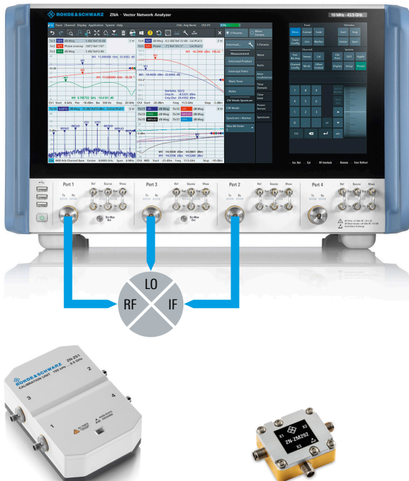
R&S®ZN-Z5x自动校准单元
