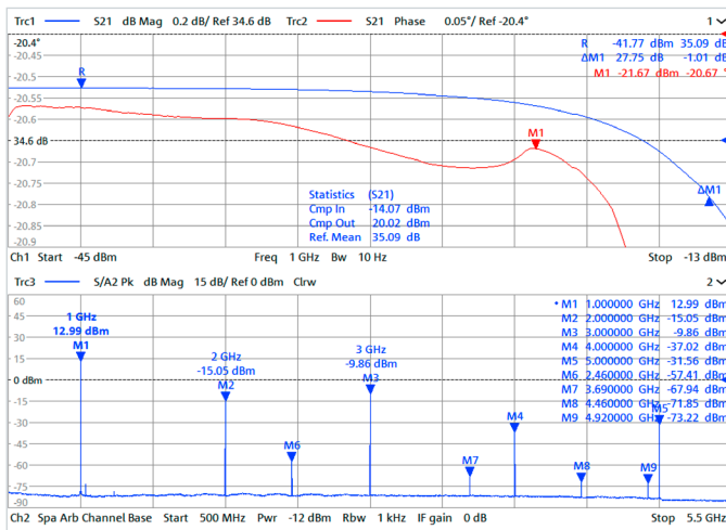
R&S®ZNA-K1频谱分析仪选件：放大器幅度和相位压缩测量（1 GHz，顶部）以及相应的谐波和杂散频谱
