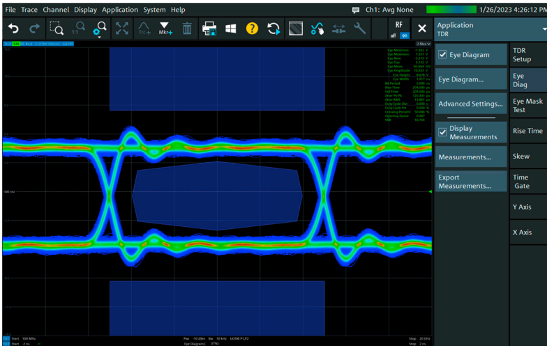
具有综合信号预失真的眼图模板测试
