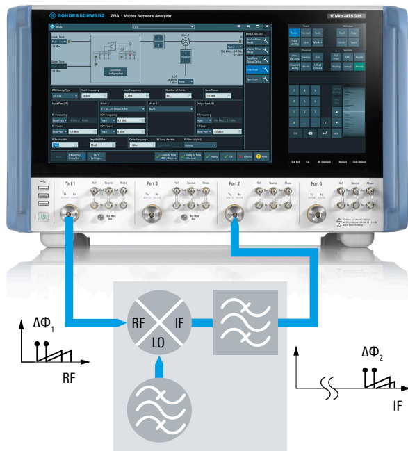
使用R&S®ZNAxx-B213内部合路器或外部合路器获得的双音信号
