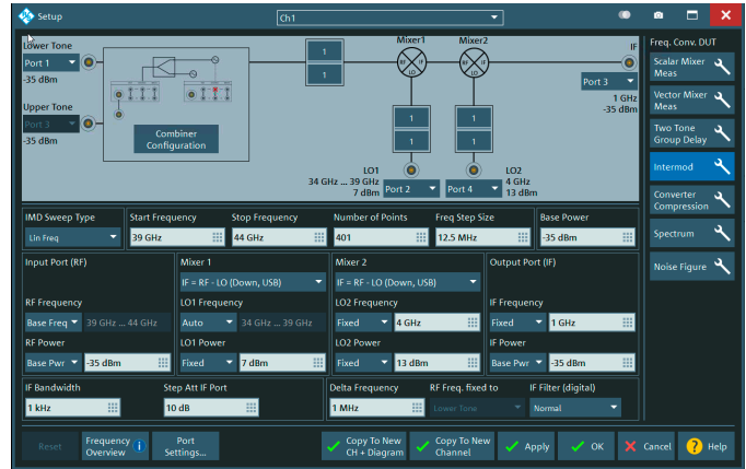
一体化对话框显示两级变频接收机的互调测量设置
