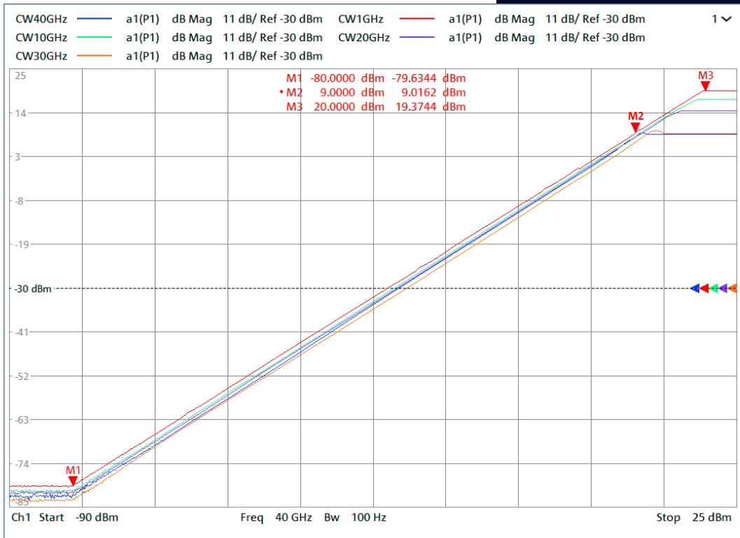
功率扫描范围高达100 dB
