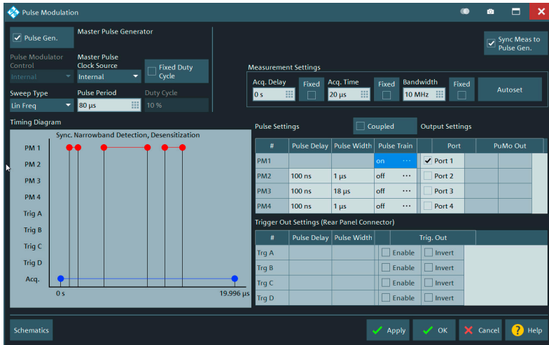
脉冲信号测量参数配置
