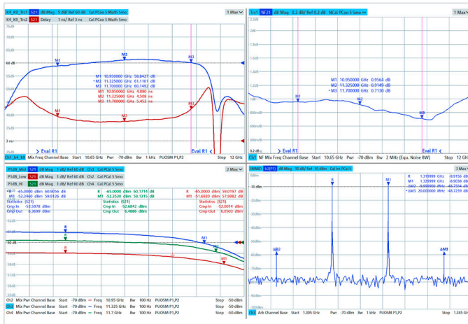
嵌入式本振变频器测试的示例结果:变频增益、群时延、噪声系数、压缩点、互调
