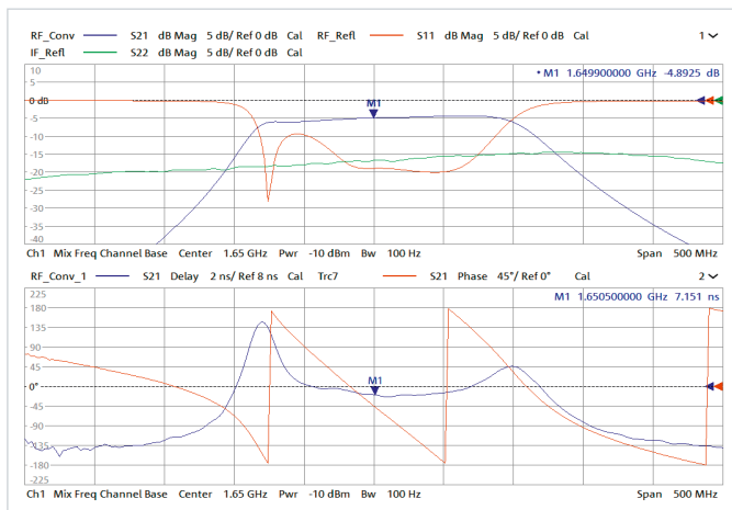
变频器测量结果包括回波损耗、变频损耗、相位和群时延
