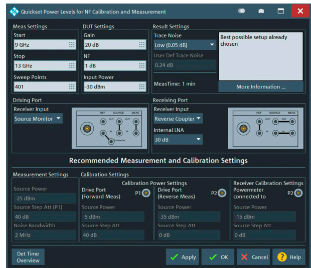
Quickset对话框用于以交互方式半自动配置合适的测试参数与R&S®ZNA硬件
