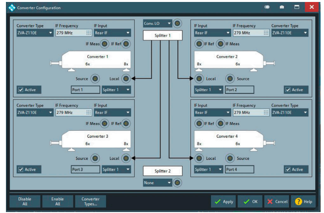
软件配置
