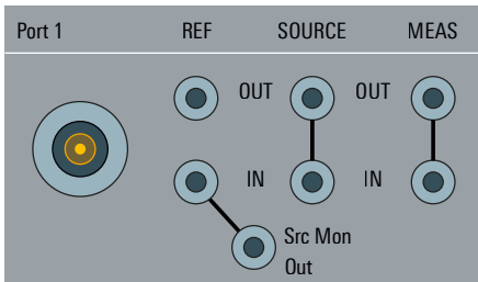
直接信号源监测接入(R&S®ZNAxx-B161/-B163)所需的R&S®ZNAxx-B16前面板跳线位置
