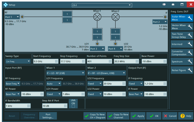
以被测设备为中心的混频器测量配置
