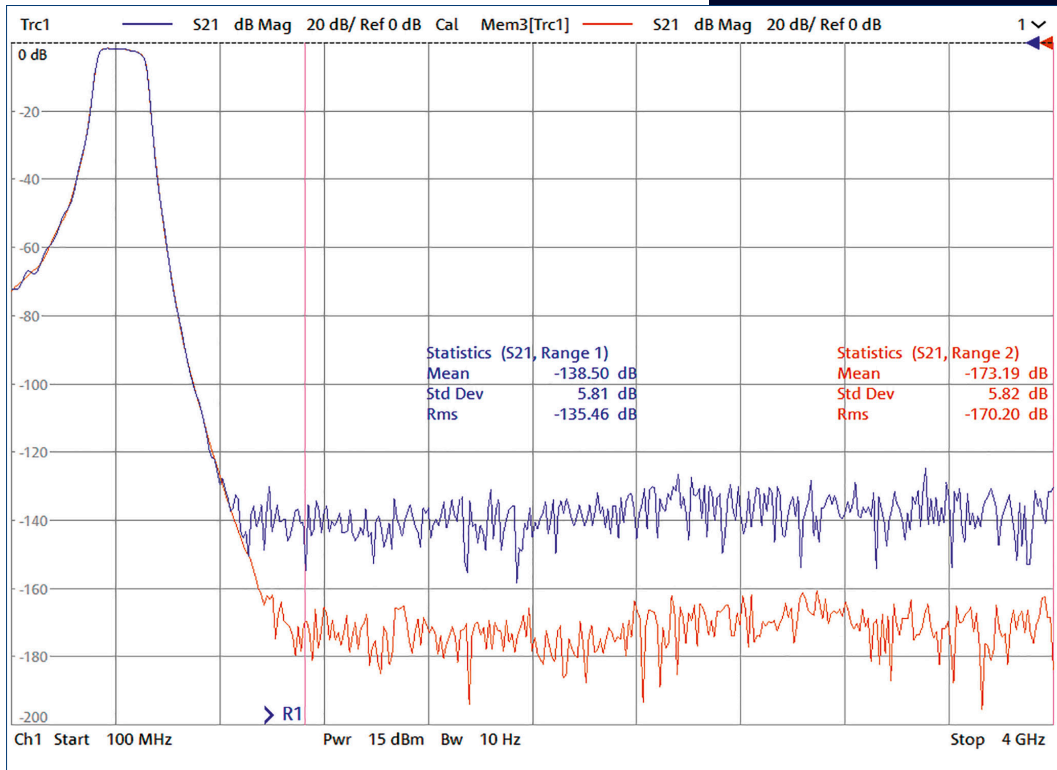
动态范围: 最大规格输出功率条件下, 无选件 (蓝色迹线: 10 Hz中频带宽时); 最大规格输出功率条件下, 反向耦合器模式, 接收机步进衰减器设为0 dB (红色迹线: 1 Hz中频带宽)
