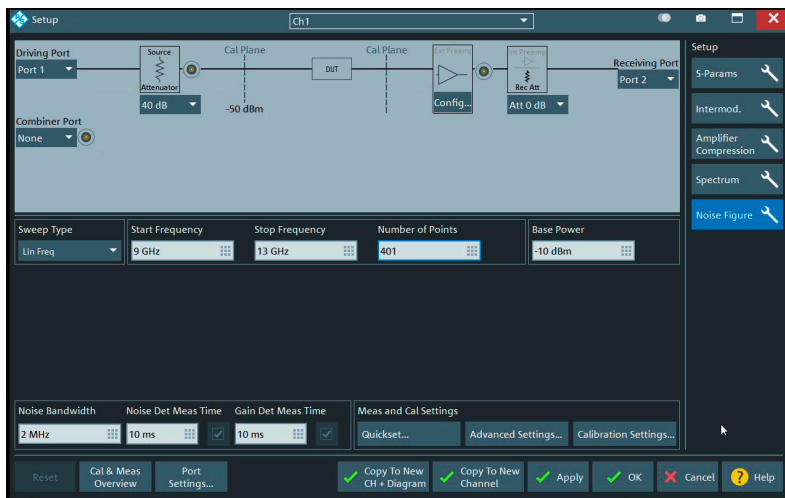
主界面用于配置放大器、混频器、变频器和收发模块的噪声系数测量
