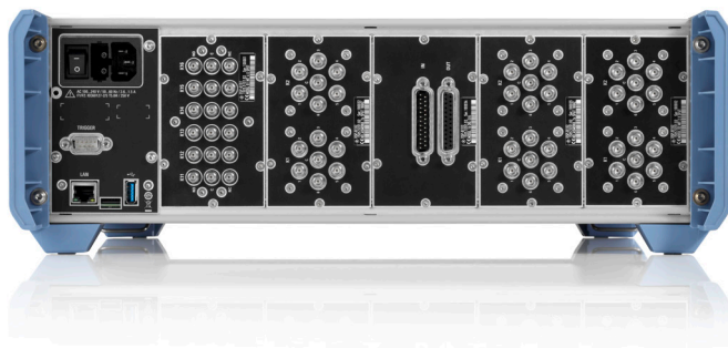
R&S®OSP320后视图
