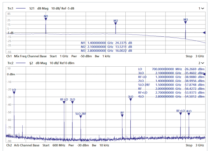
R&S®ZNA-K1频谱分析仪选件：混频器输出频谱
