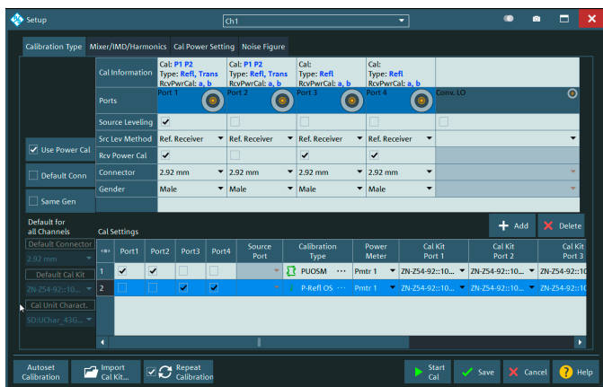
R&S®SMARTerCal结合系统误差校正、接收机功率校准和信号源绝对电平校准。
