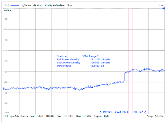
R&S®ZNA-K1分析功能：显示不同分段的功率密度比和噪声功率标记功能
