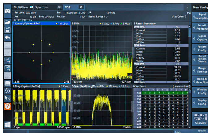
Демодуляция сигнала Bluetooth® с помощью опции R&S®FPL1-K70
