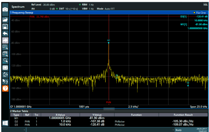
标记功能实现简单的相位噪声测量
