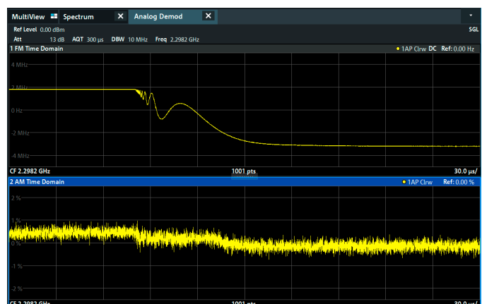
VCO切换阶段的频率和幅度的瞬态响应
