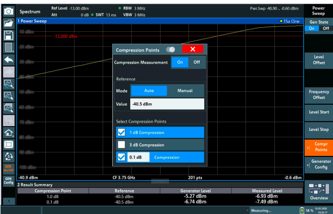
测量1 dB和0.1 dB压缩点
