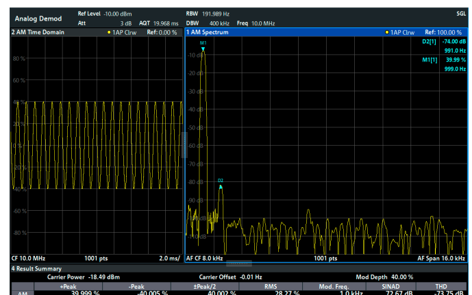
Klirrfaktormessung an einem amplitudenmodulierten Signal: Die erste Oberwelle des Modulationssignals ist mit 74 dB gut unterdrückt
