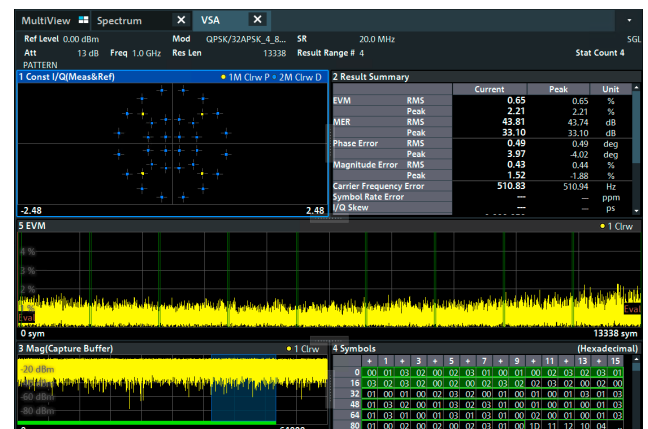
Demodulation eines DVB-SX2-Multi-Modulationssignals mit der Option R&S®FPL1-K70M (Option R&S®FPL1-K70 erforderlich)
