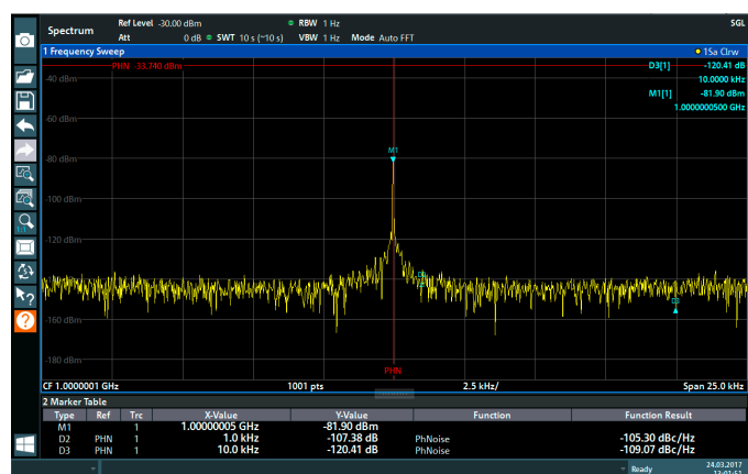
Einfache Messung des Phasenrauschens mit einer Markerfunktion
