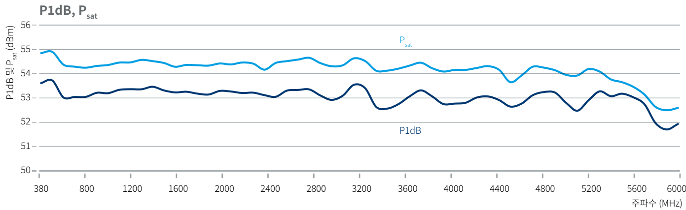
증폭기 성능 측정(R&S®BBA300-CDE180)
