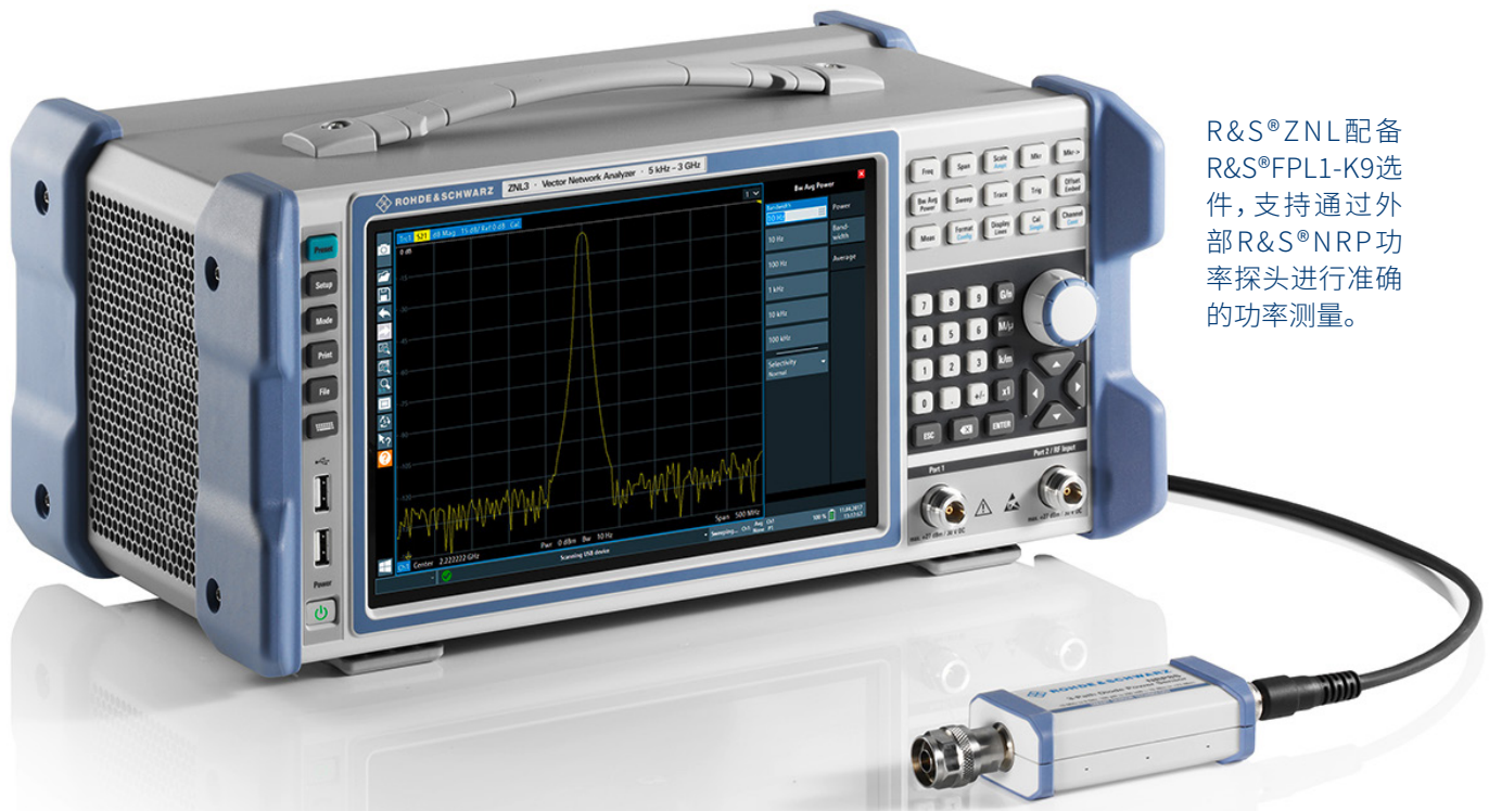
R&S®NRP 功率探头示例： R&S®NRP8SN 和 R&S®NRP8S 三通道二极管功率探头。
