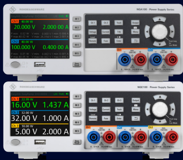
R&S®NGA142 2チャンネル電源および R&S®NGE103B 3チャンネル電源
