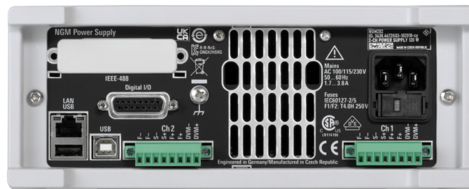
R&S®NGM202の背面図
