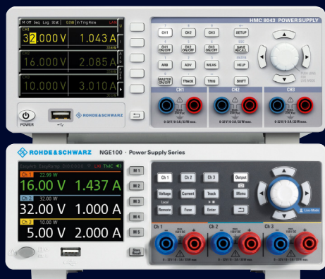
Трехканальные источники питания R&S®HMC8043 и R&S®NGE103B
