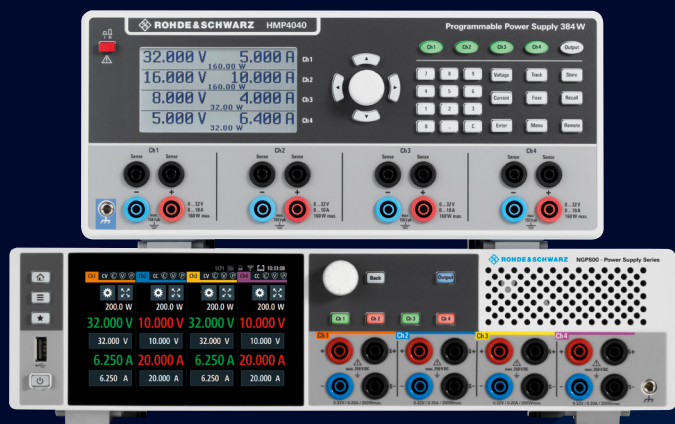
R&S®HMP4040 и R&S®NGP814 – четырехканальные источники питания
