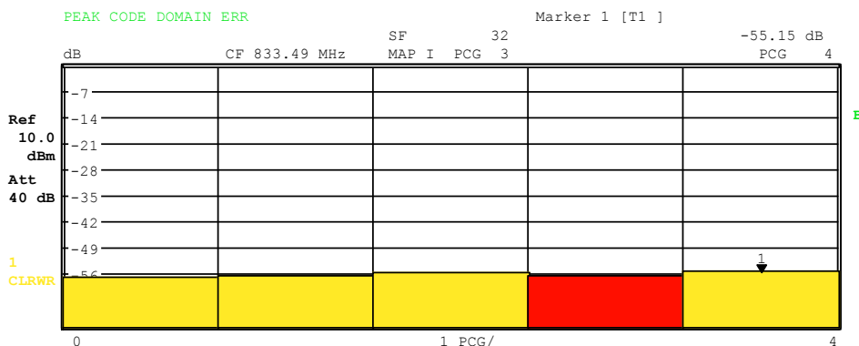
Bild 12 Peak-Code-Domain-Error für den Fall, dass alle im Signal enthaltenen Kanäle als aktiv erkannt wurden
