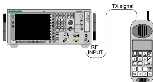
Bild 4 MS Messaufbau
