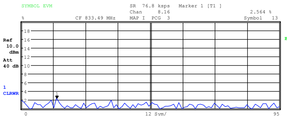
Bild 18 Error Vector Magnitude für einen PCG eines Kanals
