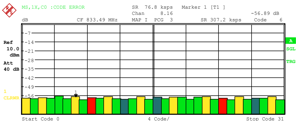
Bild 8 CDEP-Diagramm in Hadamard-Ordnung
