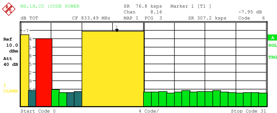
Bild 6 CDP-Diagramm in BitReverse-Ordnung für das gleiche Signal
