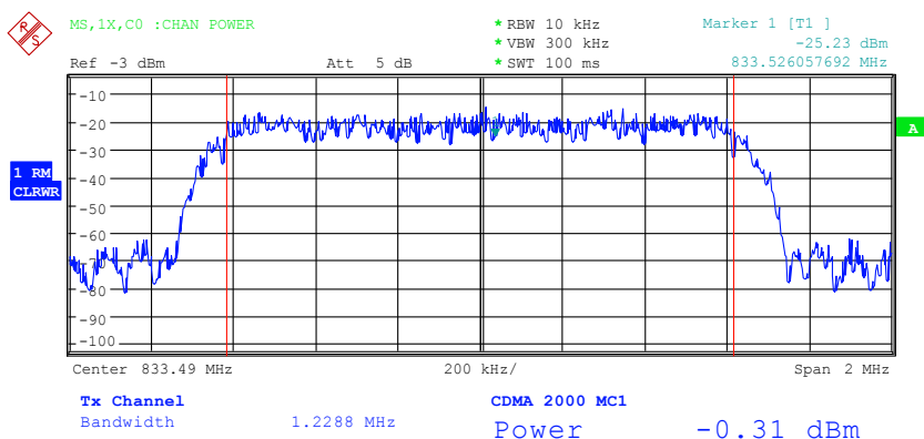
Bild 8 Messung der Leistung im 1.2288-MHz-Übertragungskanal
