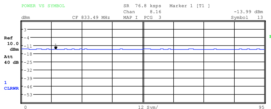
Bild 22 Power versus Symbol für einen PCG eines Kanals
