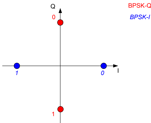
Bild 19 Konstellationsbild für BPSK-I und BPSK-Q inkl. Bitwerten
