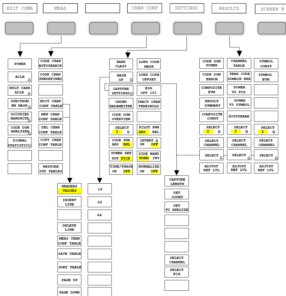
Bild 6 Übersicht der Menüs in der Applikations-Firmware R&S FS-K83
