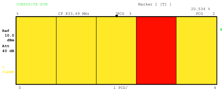
Bild 11 Darstellung des Composite EVM für den Fall, dass ein Code-Kanal nicht als aktiv erkannt wurde
