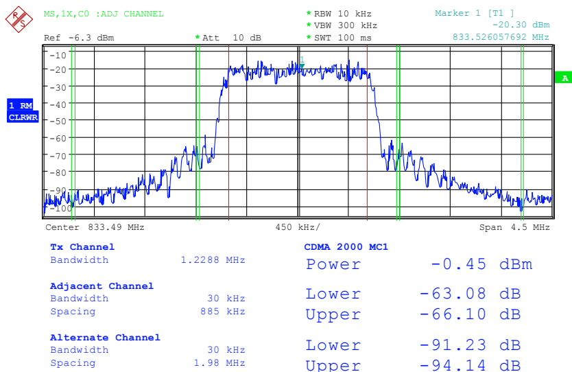
Bild 9 Messung der Nachbarkanalleistung
