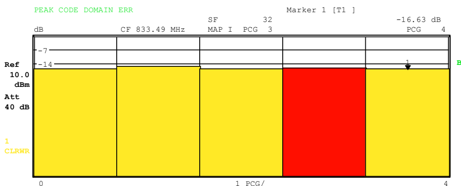
Bild 13 Peak-Code-Domain-Error für den Fall eines nicht als aktiv erkannten Kanals
