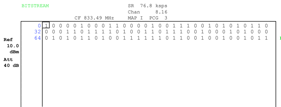
Bild 20 Demodulierte Bits für eine PCG des Kanals
