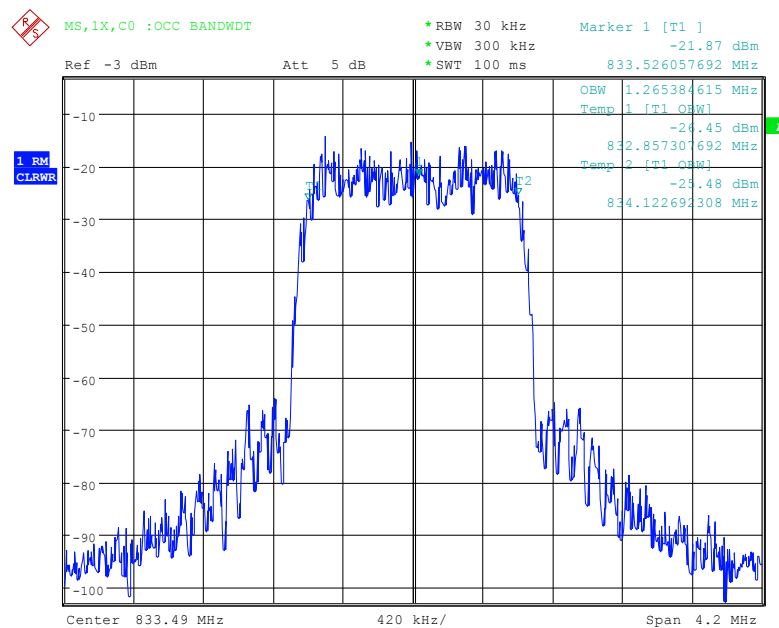
Bild 2 Messung der belegten Bandbreite
