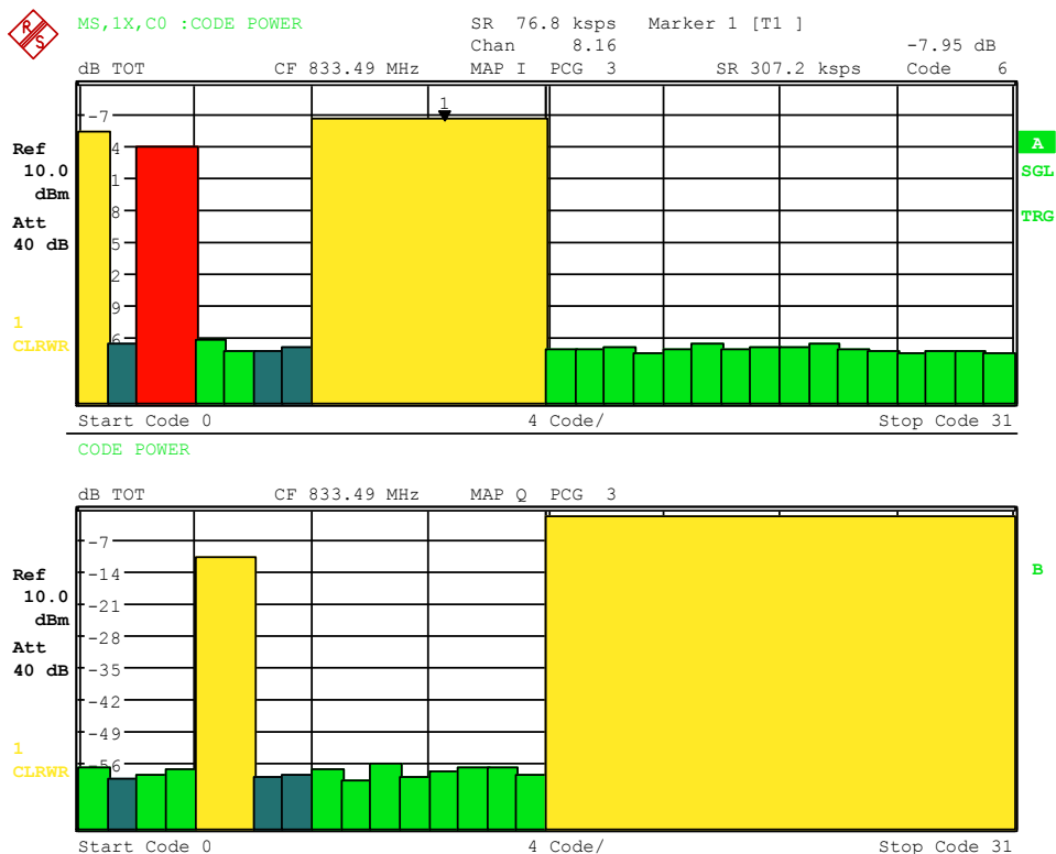
Bild 7 CDP-Diagramm in BitReverse-Ordnung im Überblicksmodus
