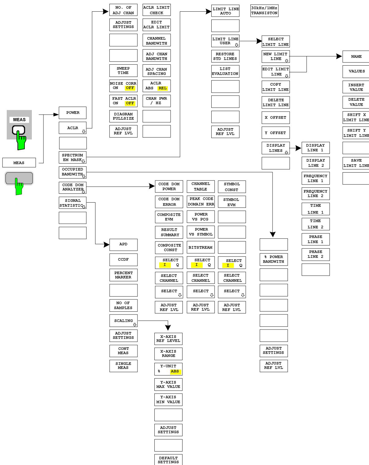
Bild 7 Übersicht der Menüs
