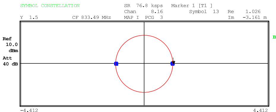
Bild 17 Symbol Constellation Diagram
