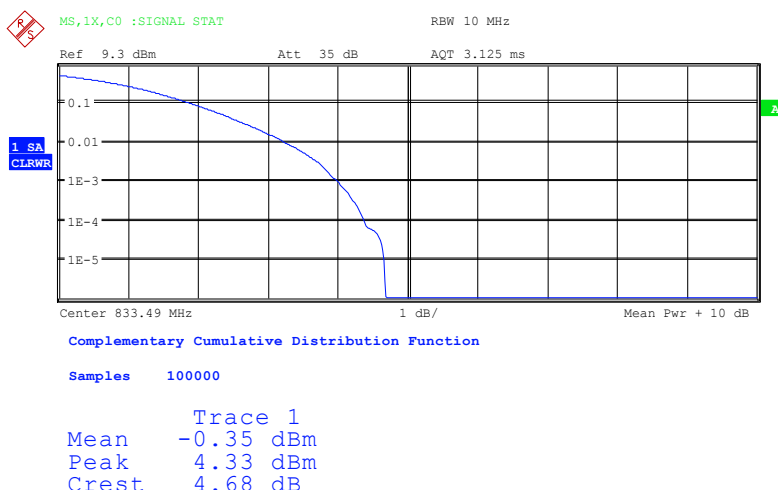
Bild 3 CCDF des cdma2000-Signals
