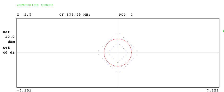
Bild 21 Composite Constellation Diagram
