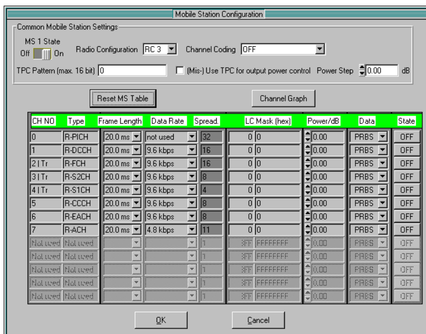
Bild 1 WinIQSIM - Mobile Station Configuration für RC 3 vor der Definition der aktiven Kanäle
