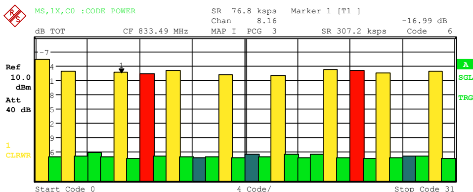
Bild 5 CDP-Diagramm in Hadamard-Ordnung
