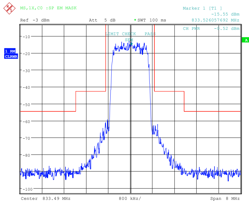
Bild 6.3-1 Messung der Spectrum Emission Mask
