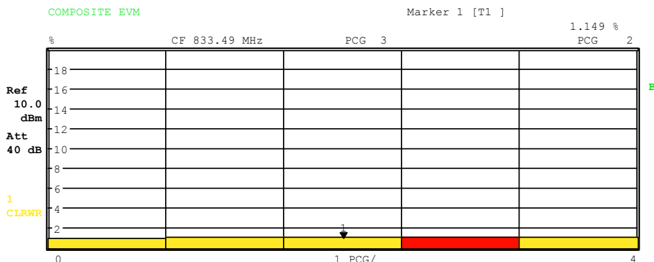
Bild 10 Darstellung des Composite EVM für den Fall, dass alle im Signal enthaltenen Kanäle als aktiv erkannt wurden
