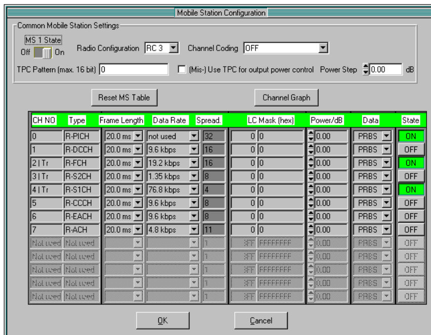
Bild 2 WinIQSIM - Konfiguration mit aktiven Kanälen
