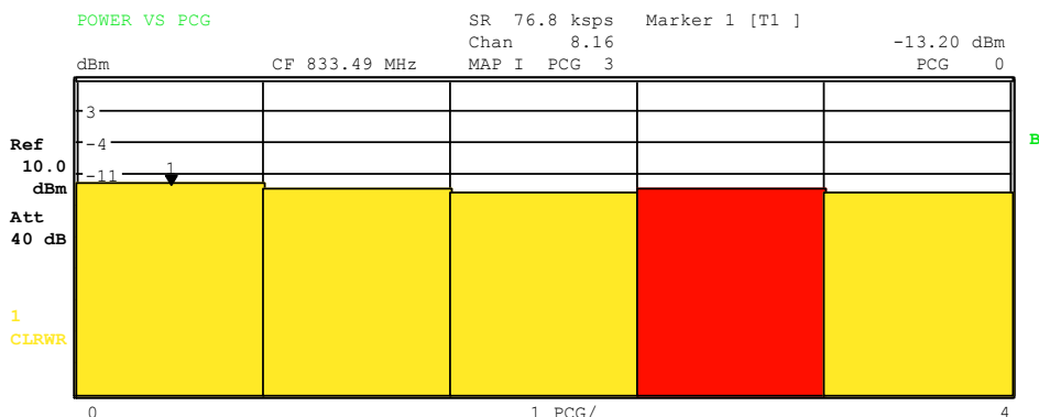
Bild 14 Power versus PCG für einen belegten Kanal mit Leistungsregelung
