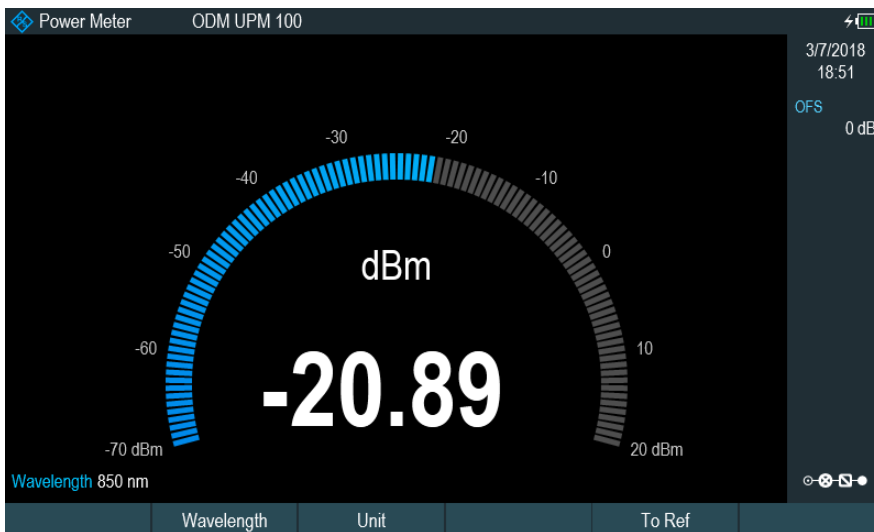
光功率测量屏幕 (R&S®FPH-K9)
