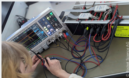
Das R&S®RTB2004 bei der Messung.
