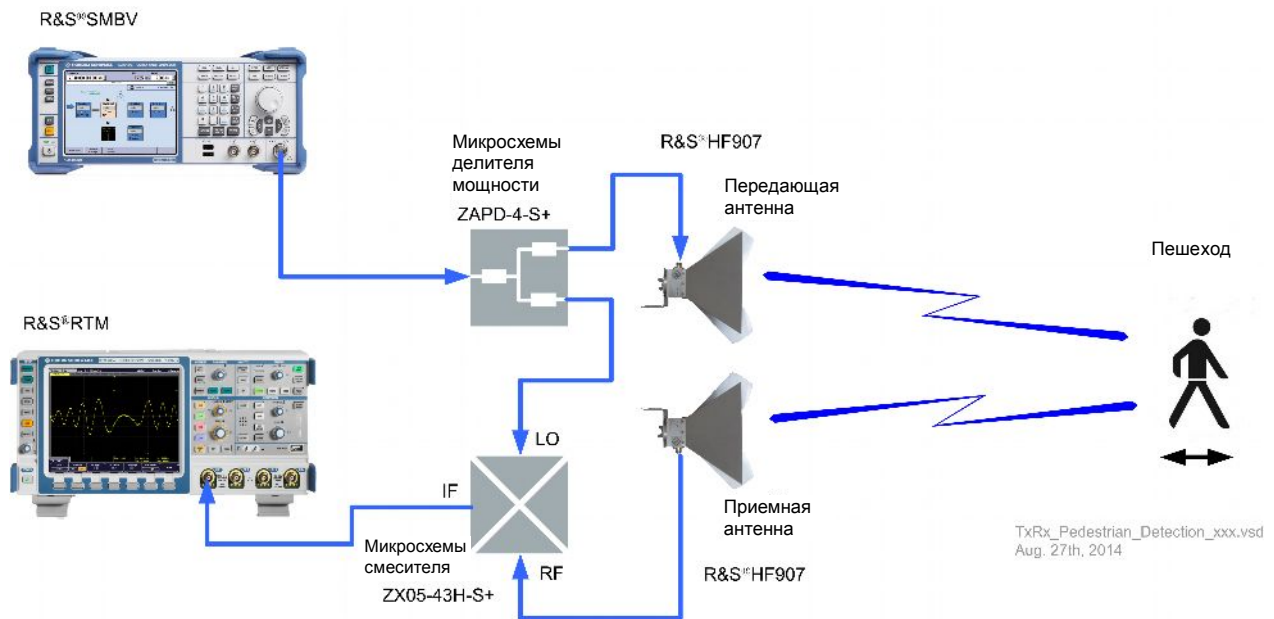
Рисунок 2-6 – Определение скорости движущихся объектов с помощью РЛС
