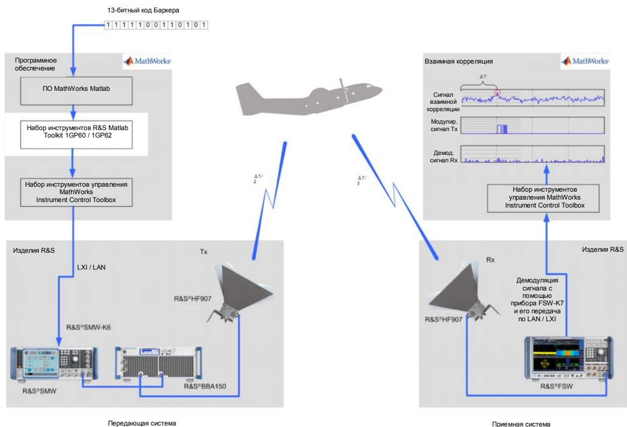
Рисунок 2-1 – Формирование и расчет характеристик модулированных сигналов с кодом Баркера
