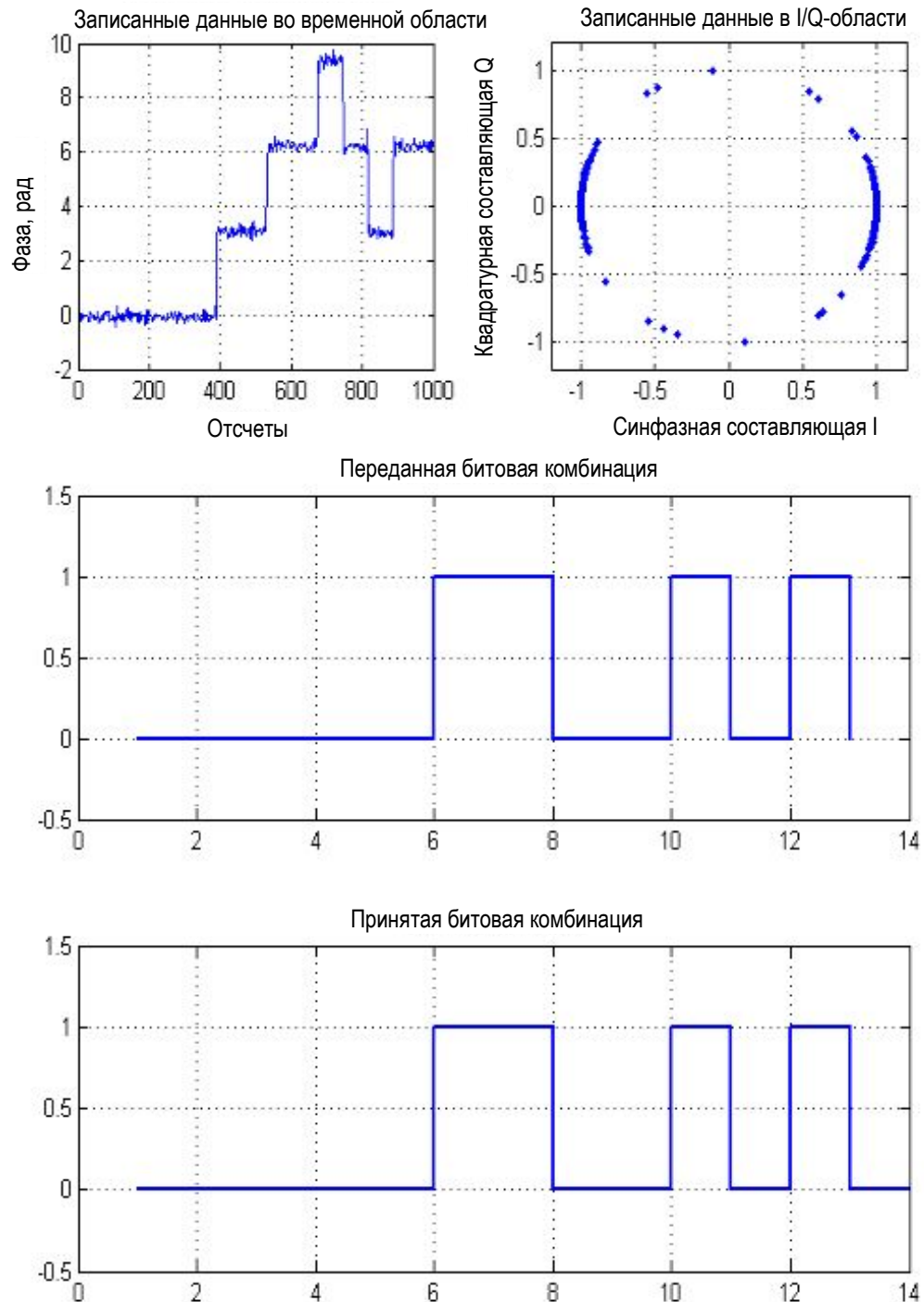
Рисунок 2-3 – Восстановление битовых данных по демодулированному сигналу
