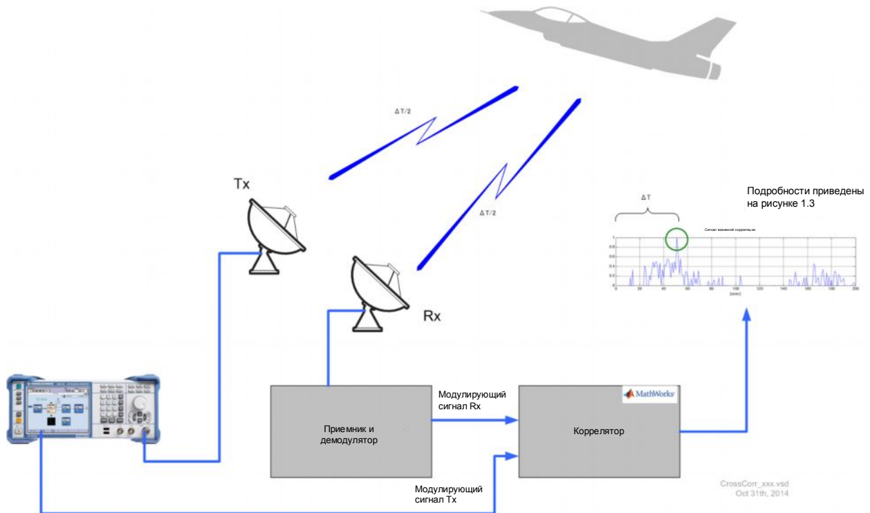
Рисунок 1-1 – Пример метода сжатия импульсов
