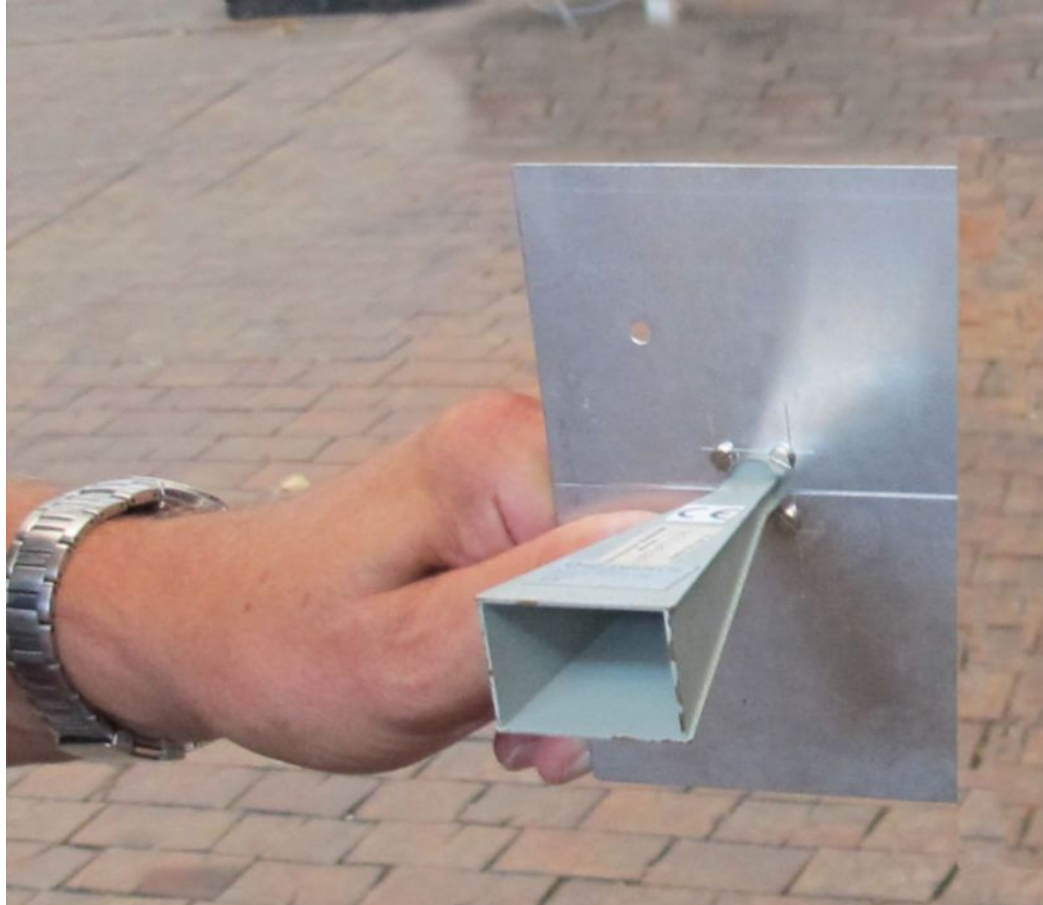
Рисунок 4-5 – Небольшая рупорная антенна, обеспечивающая усиление более чем на 20 дБи
