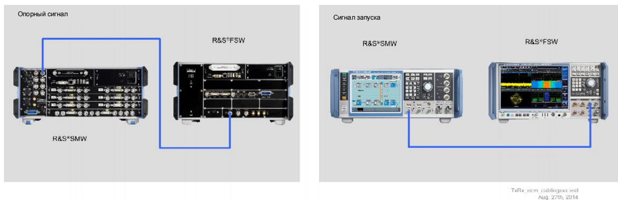
Рисунок 2-4 – Кабельные соединения для опорного сигнала и сигнала запуска
