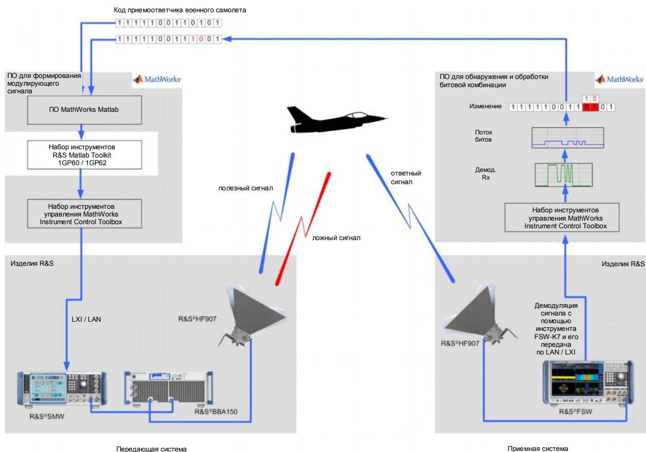
Рисунок 2-2 – Радиолокационная система с обратной связью
