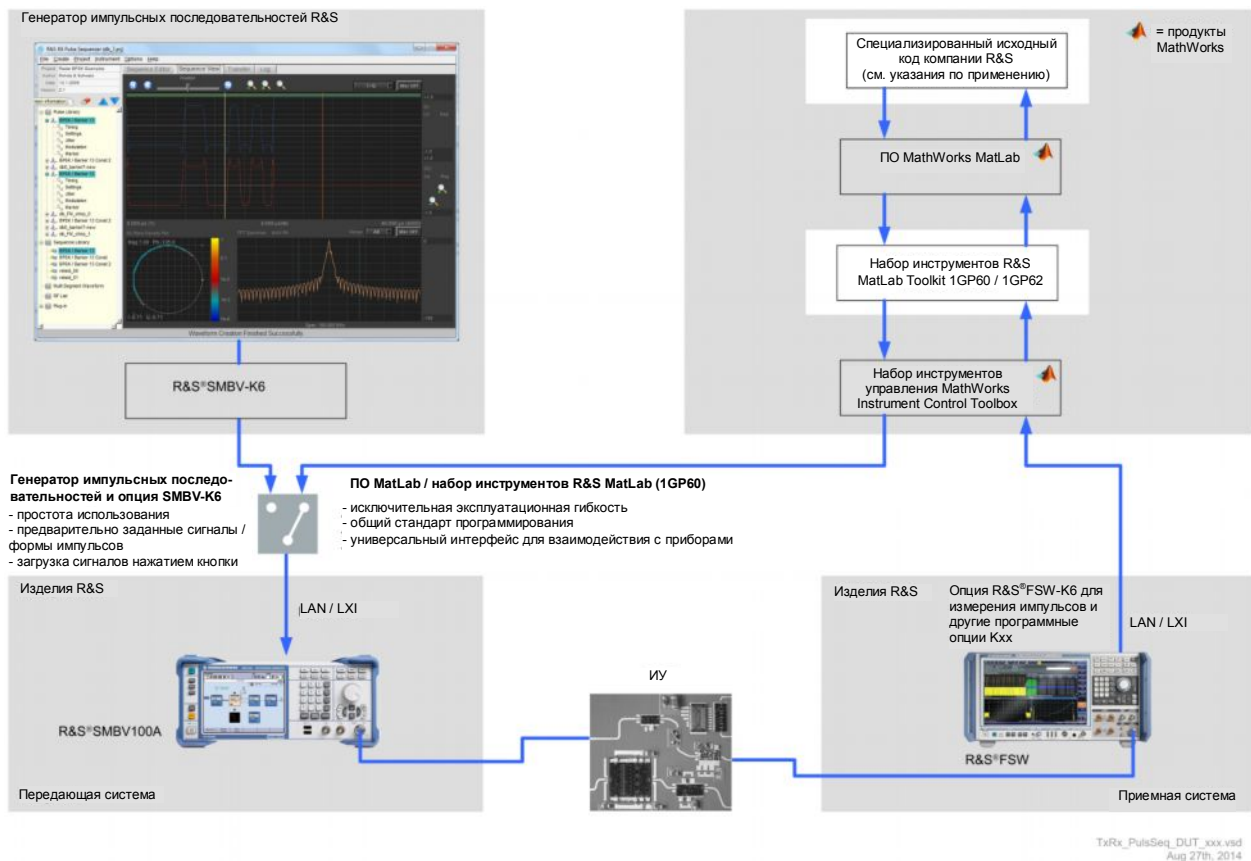
Рисунок 3-1 – Простота выбора в концепции программного обеспечения R&S для РЛС
