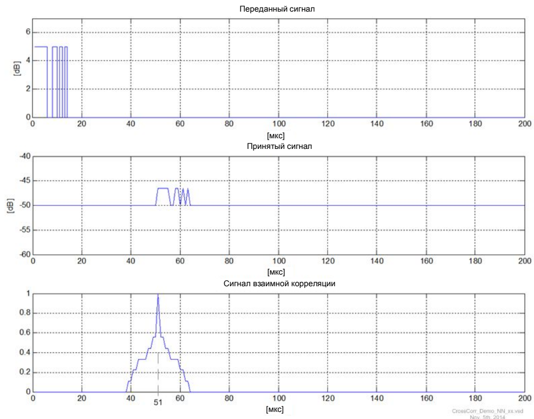
Рисунок 1-2 – Сигнал взаимной корреляции T_x / R_x с использованием кода Баркера при отсутствии шума
