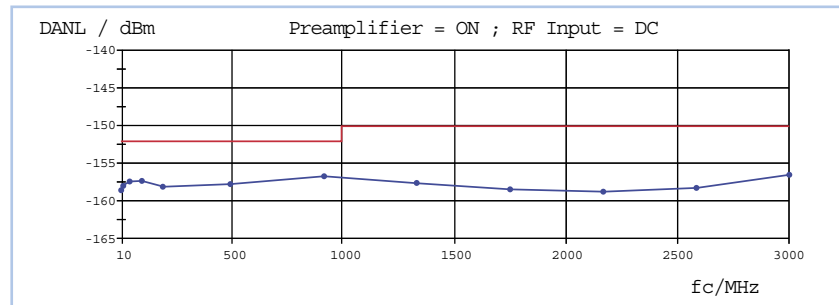
Beispiel aus Typprüfungsprotokoll mit DANL
