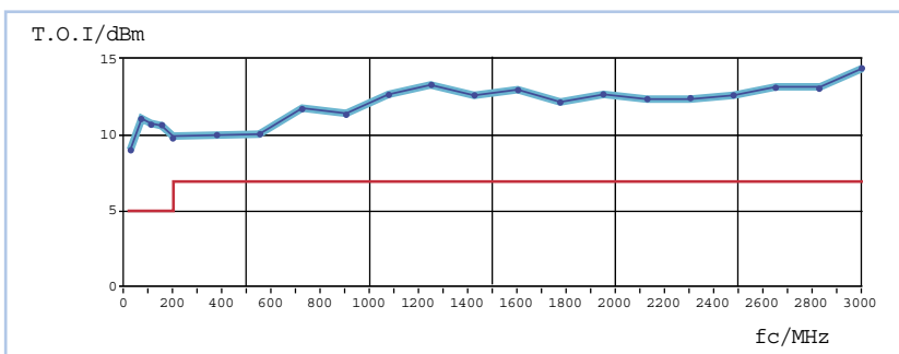
Beispiel aus Typprüfungsprotokoll mit IP3
