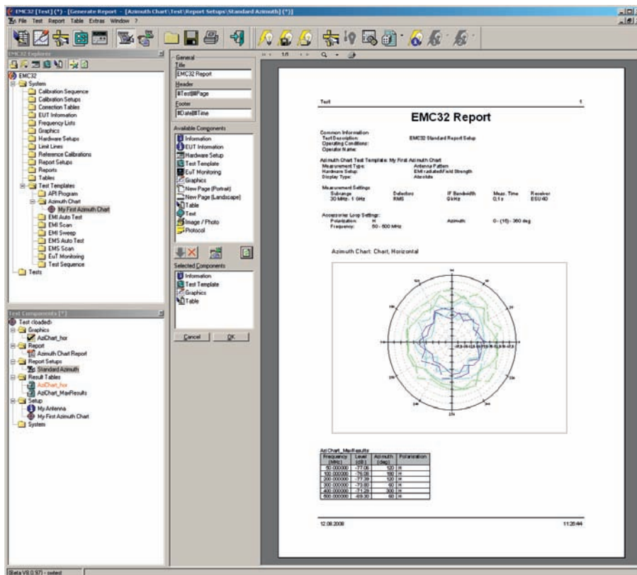
R&S®EMC32-Testreport mit Polardiagramm der Abstrahlcharakteristik
