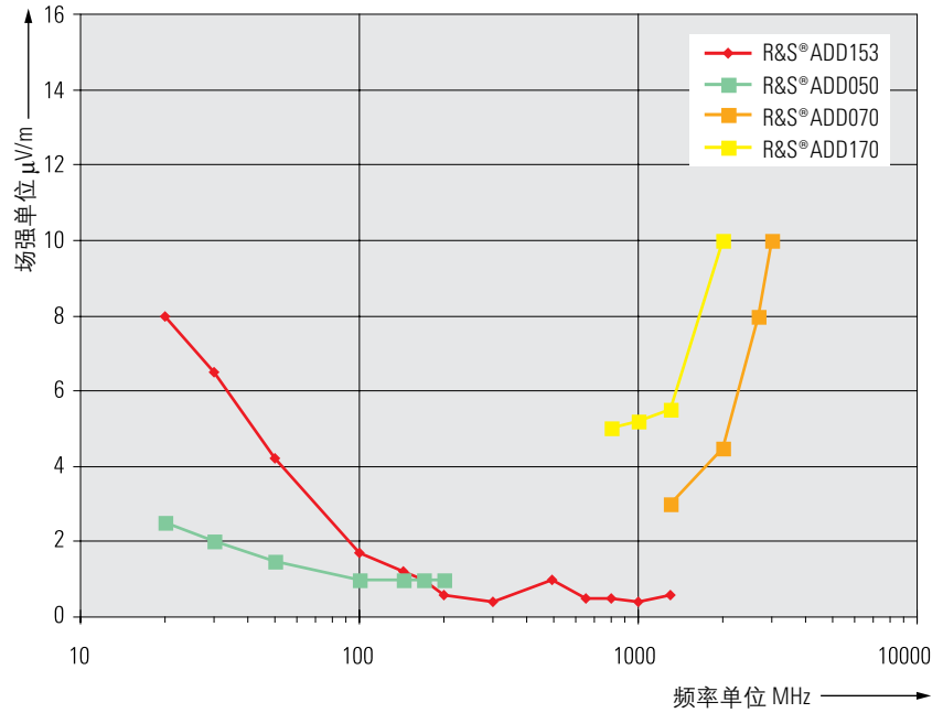
测向天线的灵敏度；平均时间1 s，方向波动 <math>2^\circ</math> RMS, 带宽1 kHz
