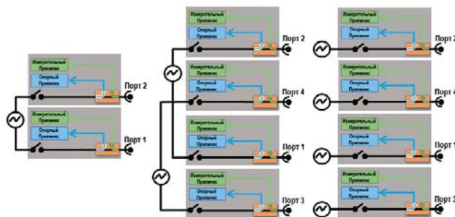
Варианты исполнения базовых блоков R&S®ZVA
