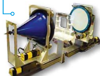
Зонды для диэлектрических измерений твердых материалов, порошков и жидкостей
