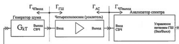
Рисунок 1б. Измерение суммарного коэффициента шума четырехполюсника и анализатора спектра KШ_{чп+вас}
