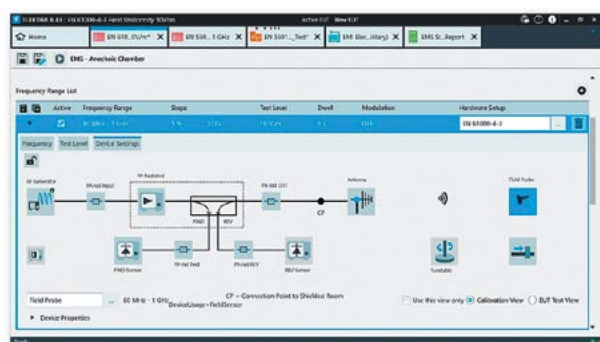
Шаблон автоматического проведения испытаний на ЭМВ с возможностью просмотра и изменения аппаратных настроек и конфигураций в одном окне
