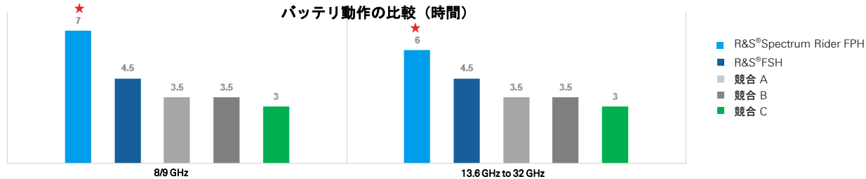
バッテリー動作の比較 (時間)
