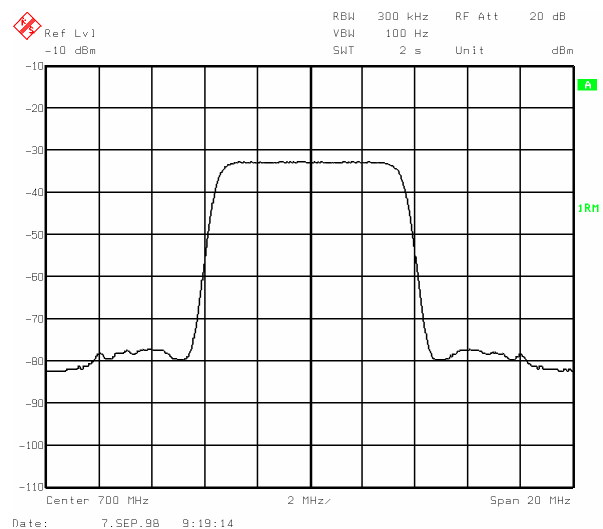
Fig. 5 PRBS spectrum
