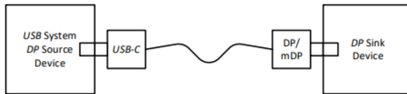
Scenario 2a Cable Wiring
