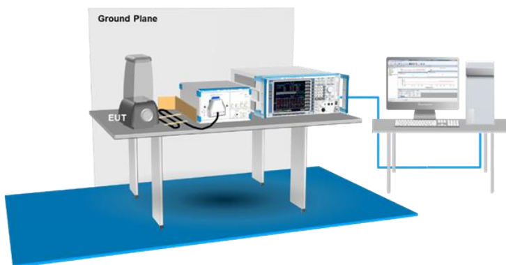
Fig. 1 EUT setup
