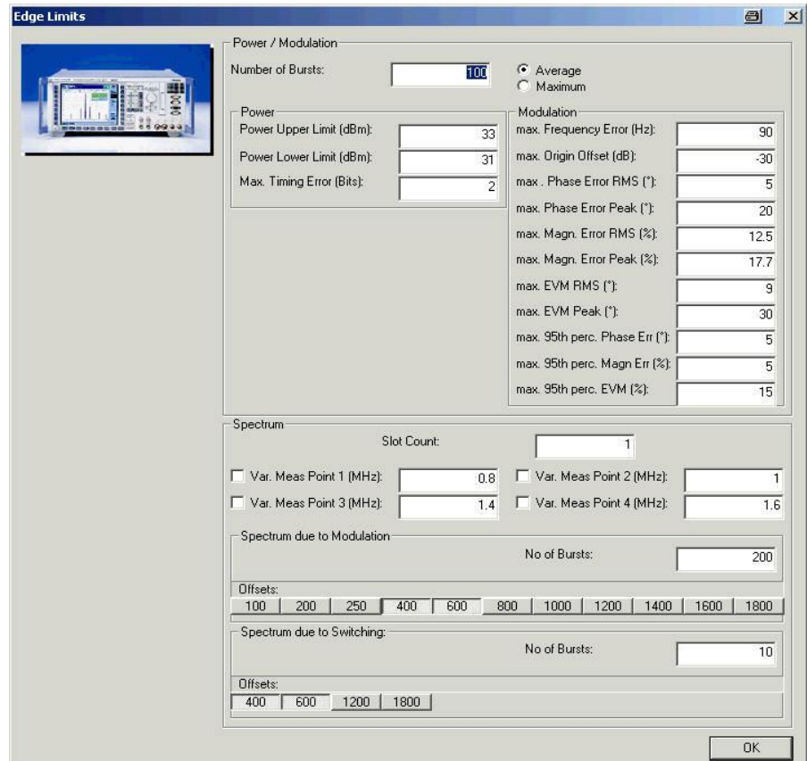
Fig. 41 - GSM Call Edge Limits
